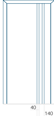
Technický výkres
